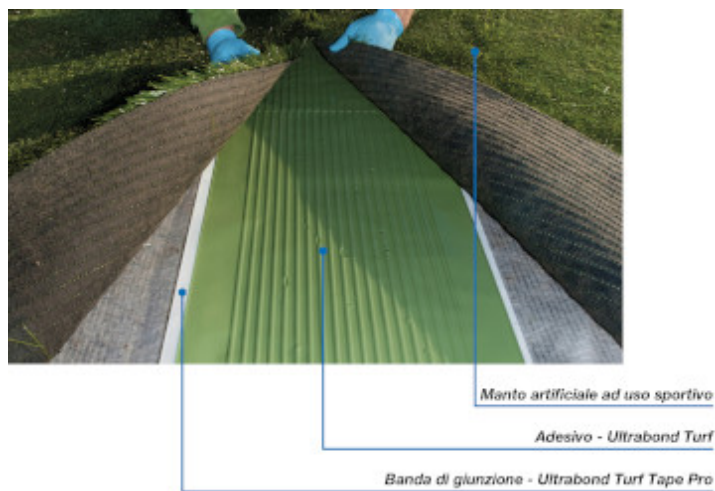
Εικ.1 - Σύστημα συγκόλλησης 3 στοιχείων: τεχνητός χλοοτάπητας, ταινία συγκόλλησης και κόλλα.
